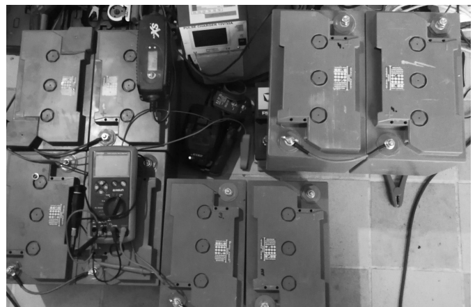
6V110Ah-s munkaakkumulátorok: ebből 2 sorba kötve 12 V, 4 pedig 24 V-os rendszert tud sok órán át kiszolgálni.
